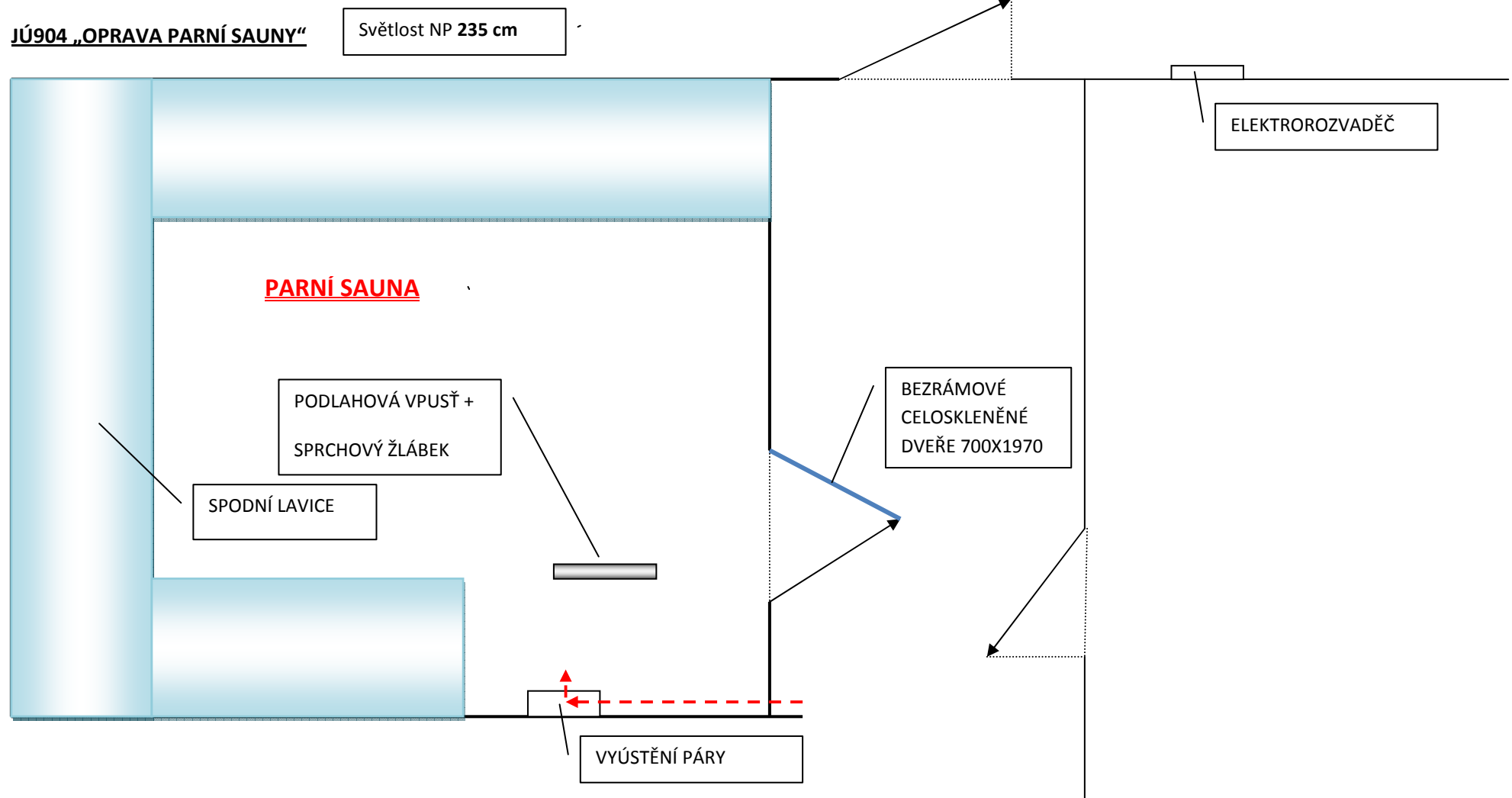
Schéma parní sauny varianta I.
